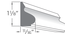
Base Cap AZM-164
